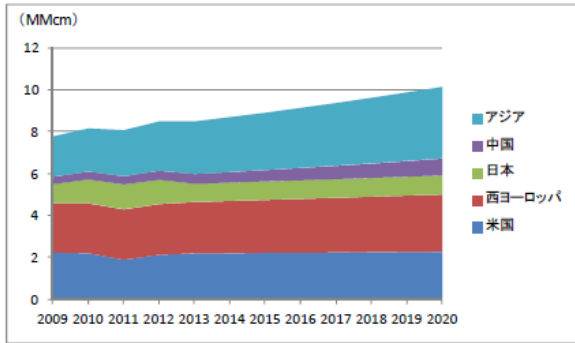
図 リークテスト向けヘリウム消費量の見通し
